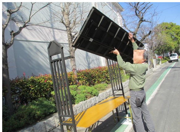
④屋根を乗せます。 ※屋根を広げ平板状にし上に乗せます (通常 2名で行います)
