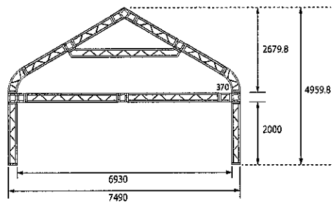
正面図
