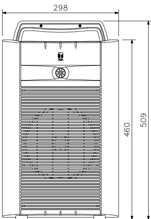
正面図
