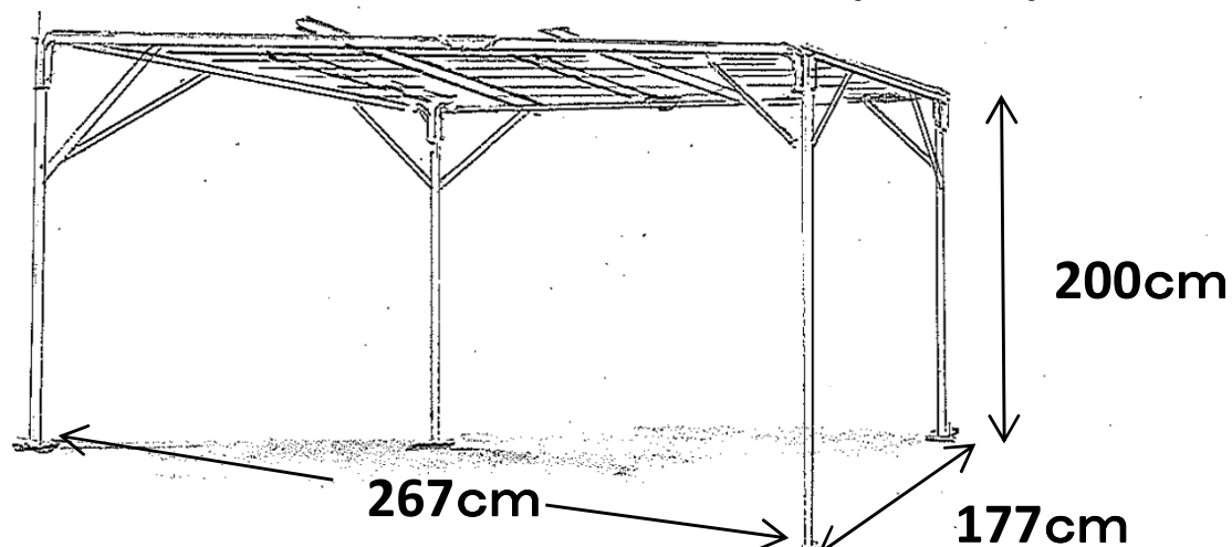
よしずテント 1.5K×2K 約3坪(9.48㎡)
