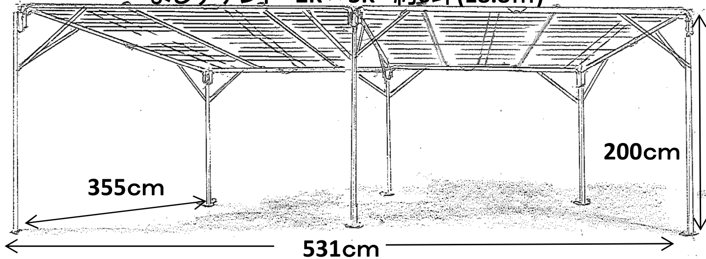
よしずテント 2K×3K 約6坪(18.8㎡)
