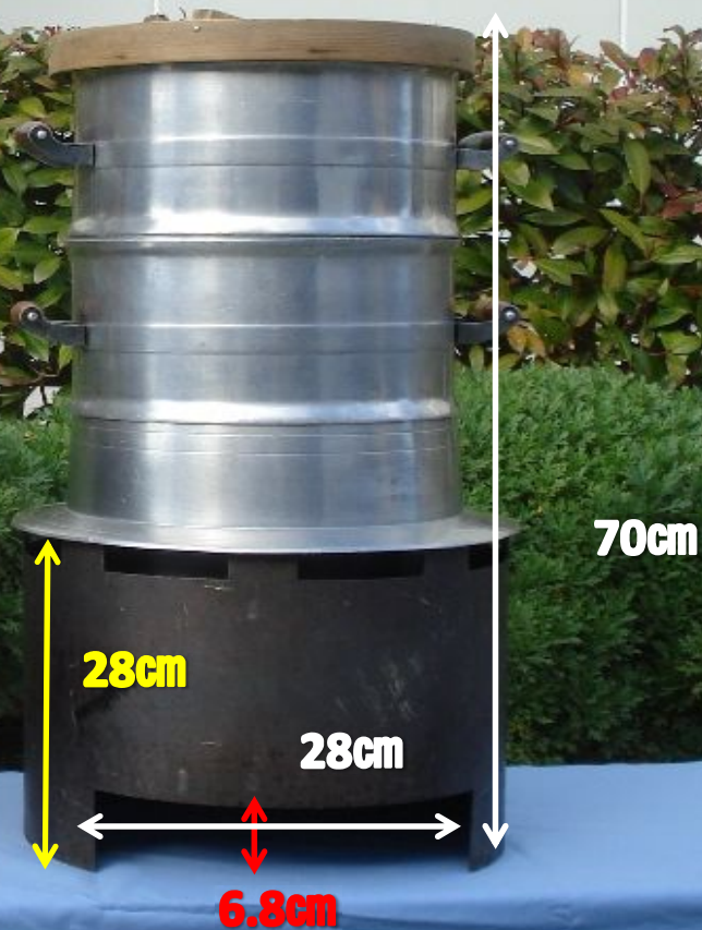
LPガス用釜戸
