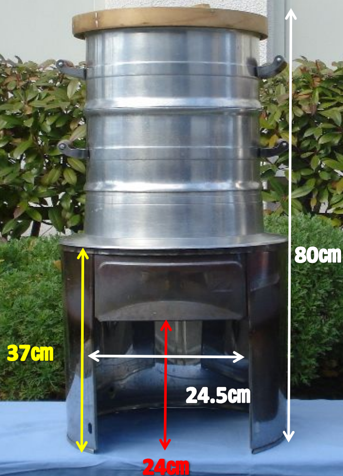
LPガス用釜戸
